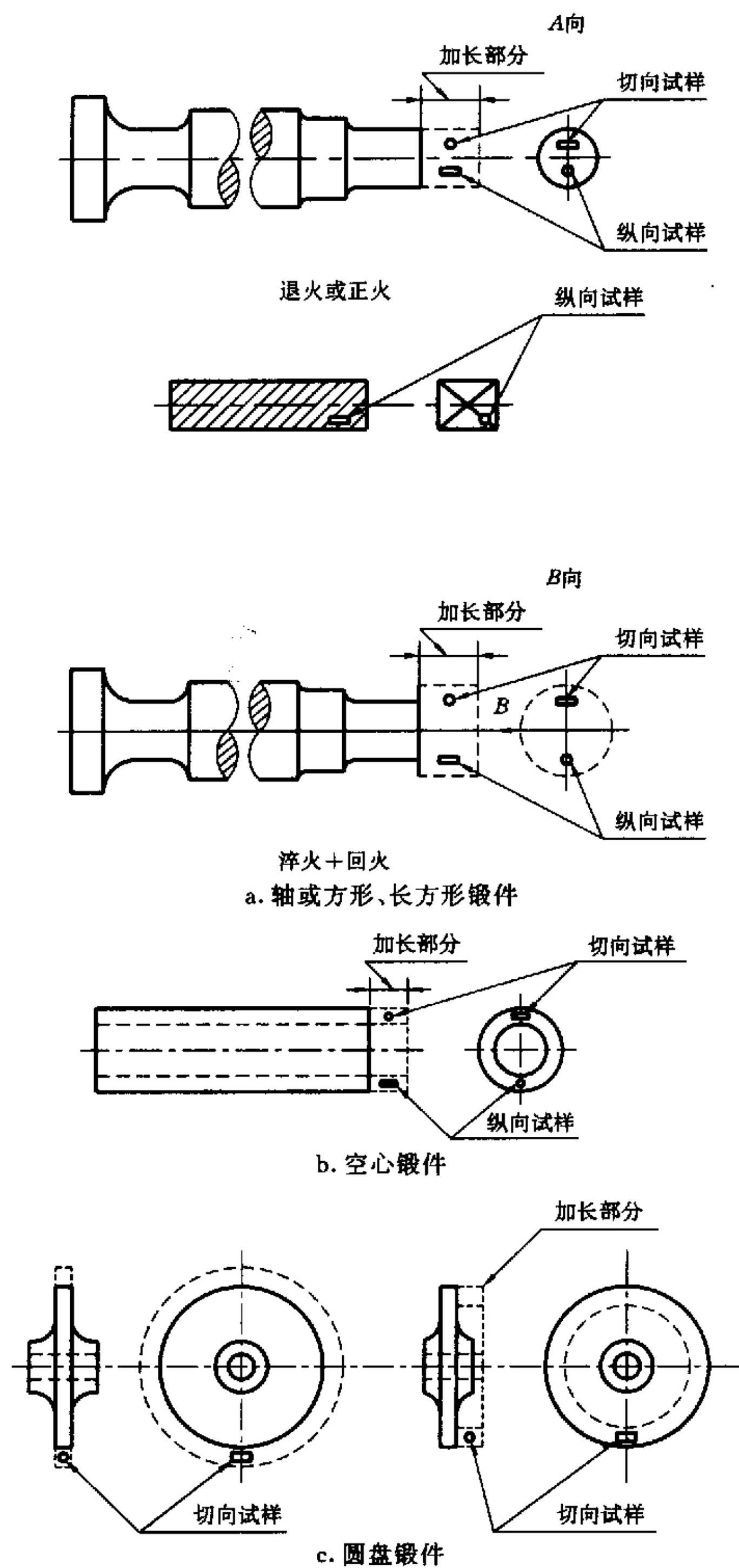
图 1 各类锻件的取样位置
