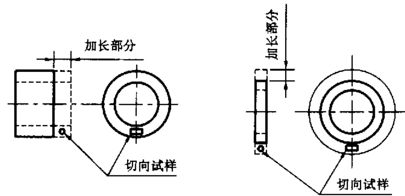
d. 环形锻件
